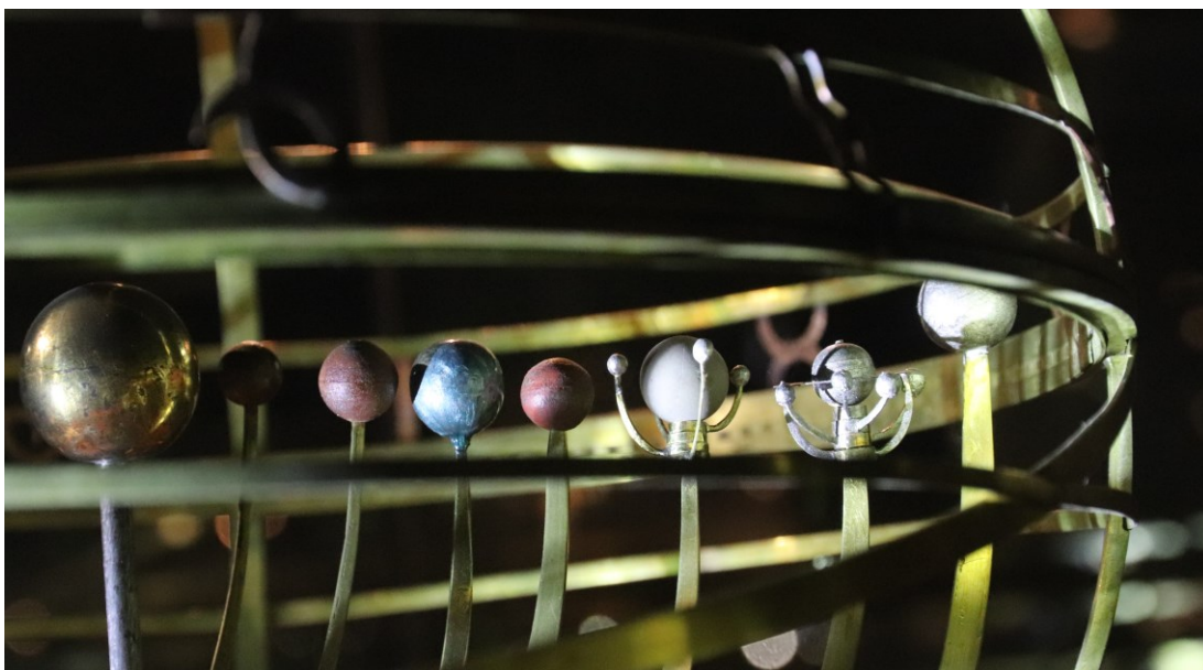
Obrázek č. 33 – Planety koperníkovského modelu
